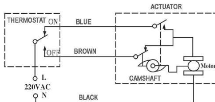
Figura 3: Desen tehnic al unei ventil de deviere cu 3 căi
