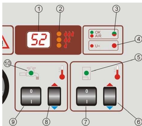
Segment din panoul de comandă
