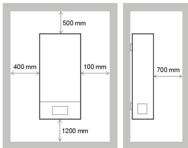
Distanță minimă la asamblare
